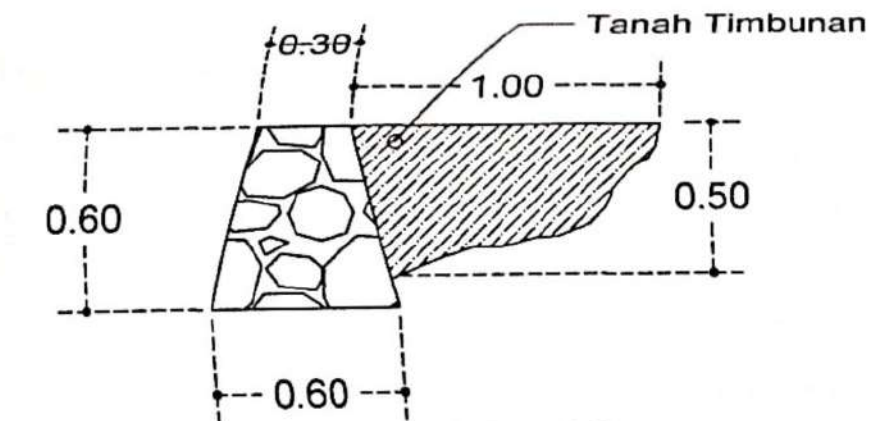
Pasangan Batu Tipe 1 P = 33 m
