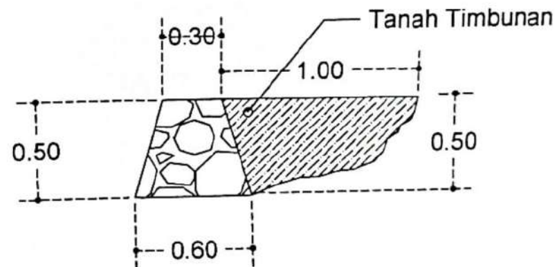
Pasangan Batu Tipe 2 P = 17 m
