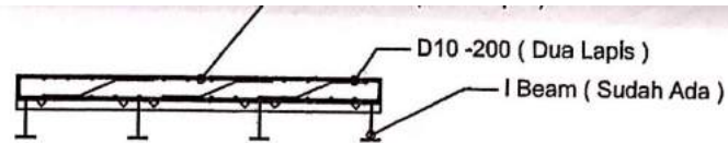
Detail Pembesian Plat Lantai Melintang Skala 1;100
